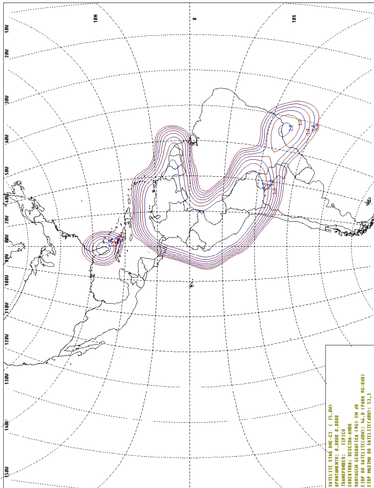
Figura 4 – Cobertura Típica de Descida do Feixe ANDK do Satélite Star One C3 (EIRP)
