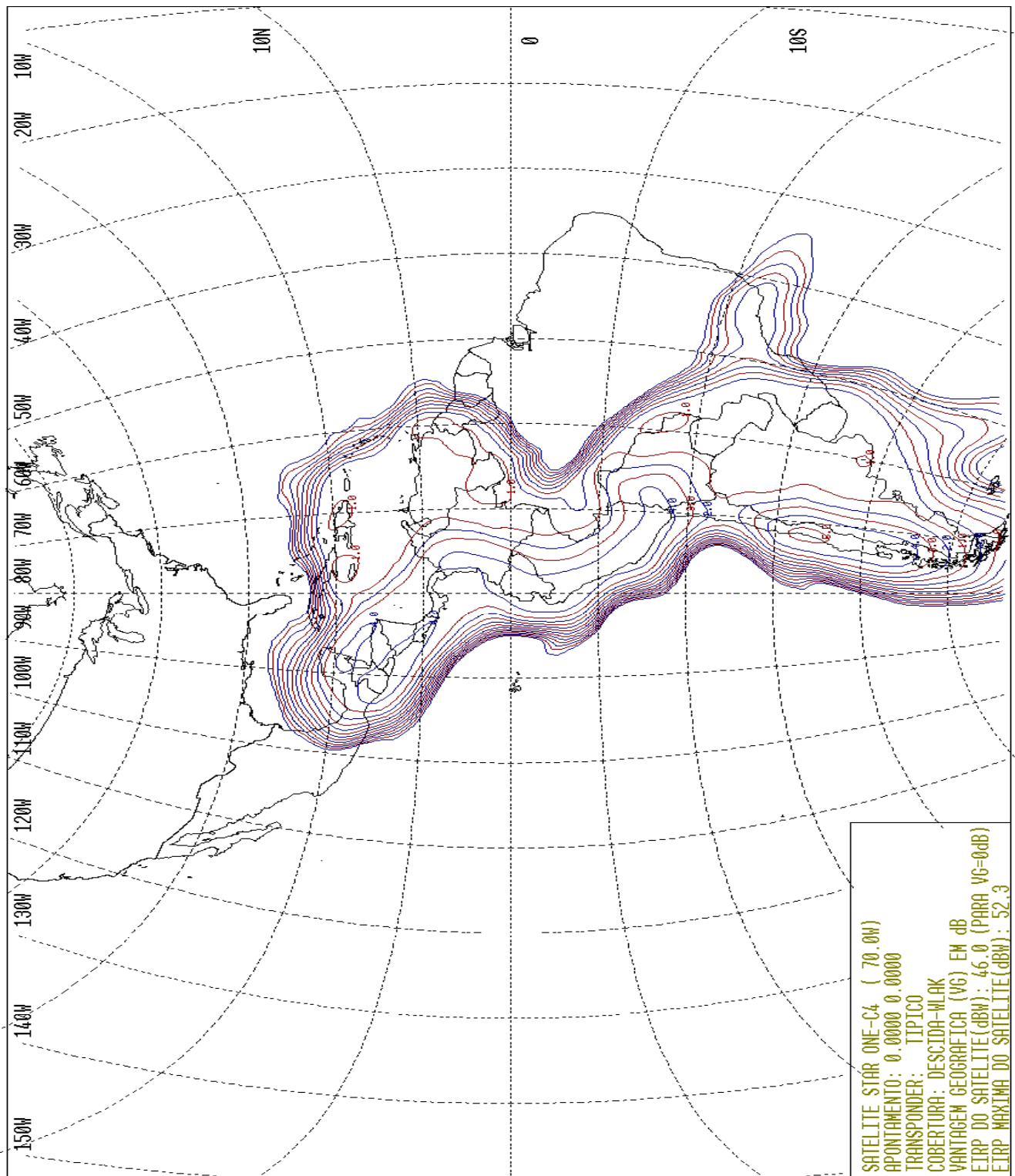
Figura 7 – Cobertura Típica de Descida do Feixe WLAK do Satélite Star One C4 (EIRP) – Vista Hemisférica
