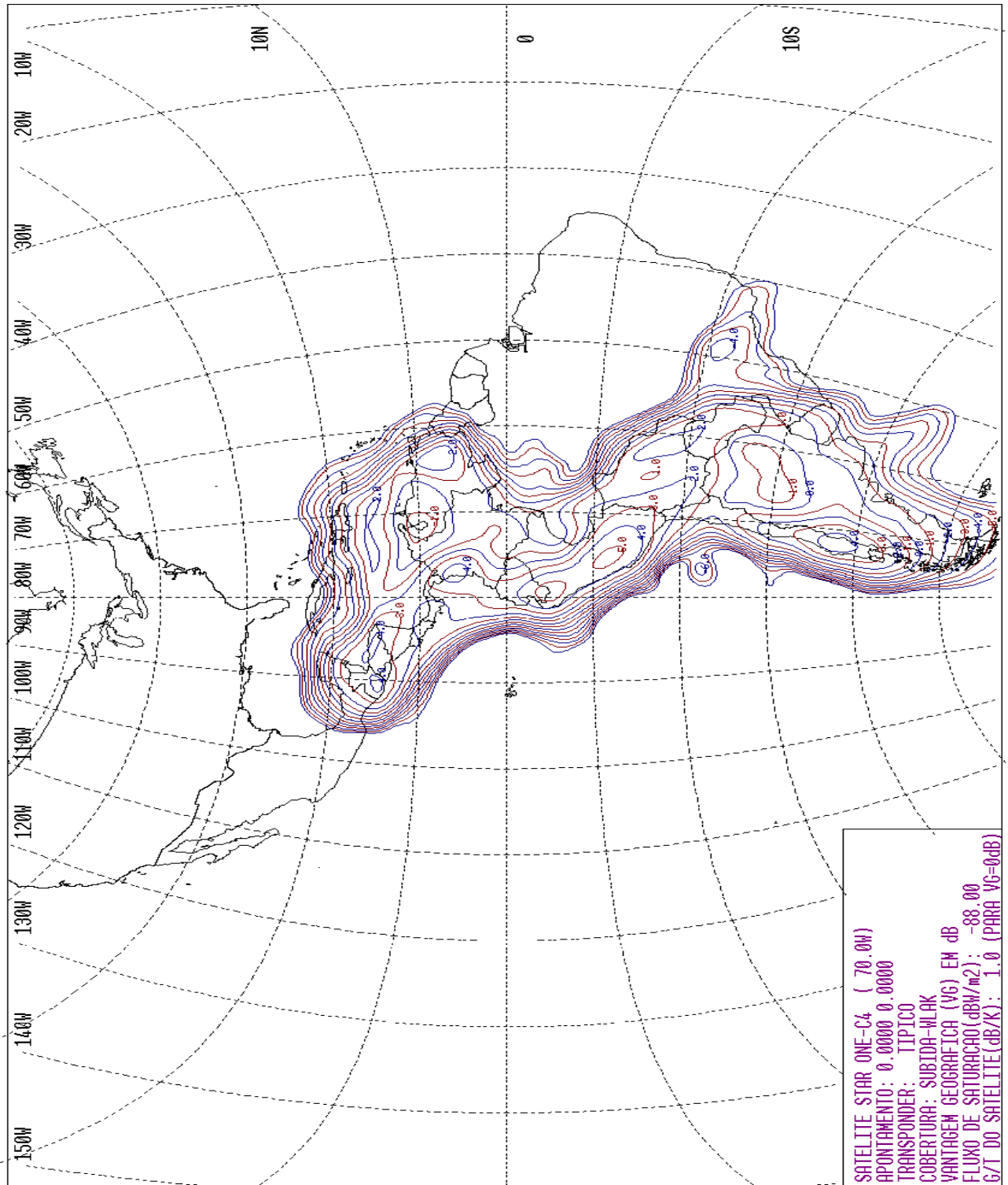
Figura 5 – Cobertura Típica de Subida do Feixe WLAK do Satélite Star One C4 (G/T) – Vista Hemisférica
