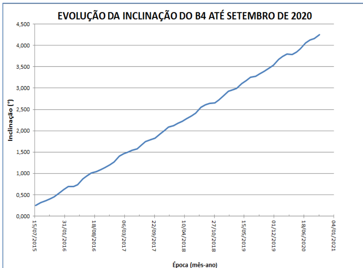
Figura 4 – Evolução da Inclinação da Órbita do Satélite Brasilsat B4
