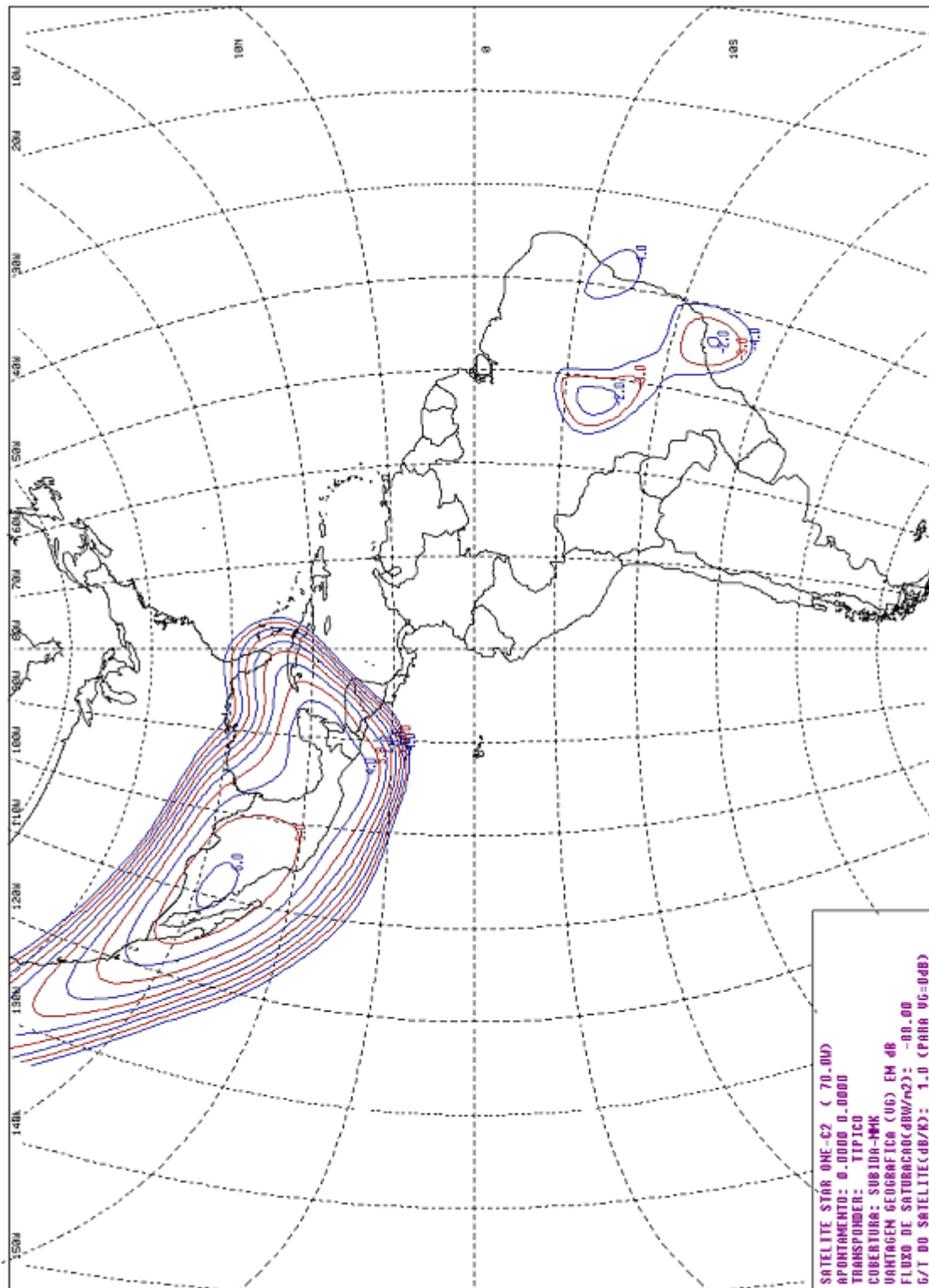
Figura 3 – Cobertura Típica de Subida do Feixe MMK do Satélite Star One C2 (G/T) – Vista Hemisférica
