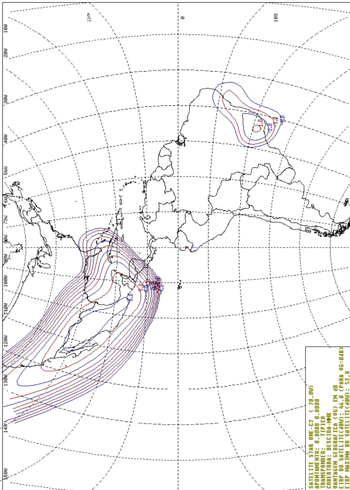
Figura 5 – Cobertura Típica de Descida do Feixe MMK do Satélite Star One C2 (EIRP) – Vista Hemisférica
