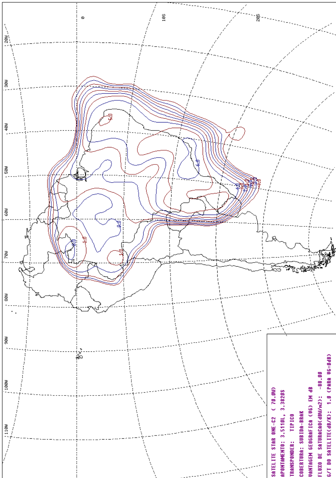
Figura 1 – Cobertura Típica de Subida do Feixe BRAK do Satélite Star One C2 (G/T)
